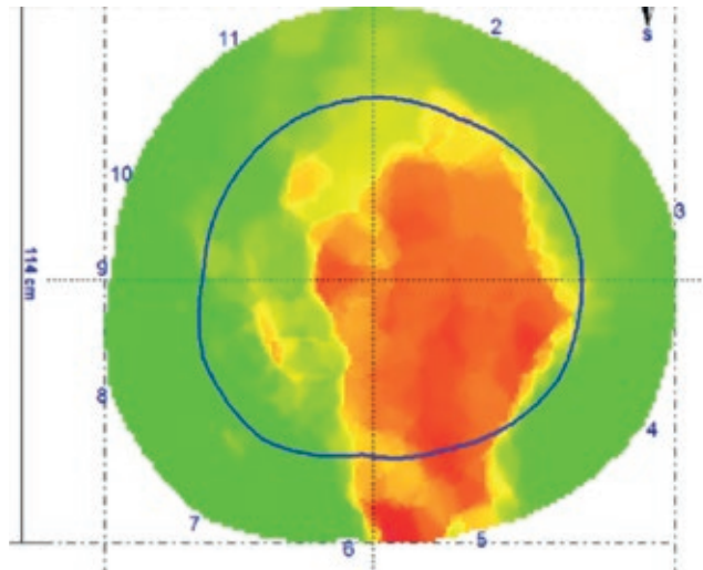
Analyse des Baumstammes mit Schalltomografie: Der rote Bereich zeigt die Schwächung des Holzkörpers.
